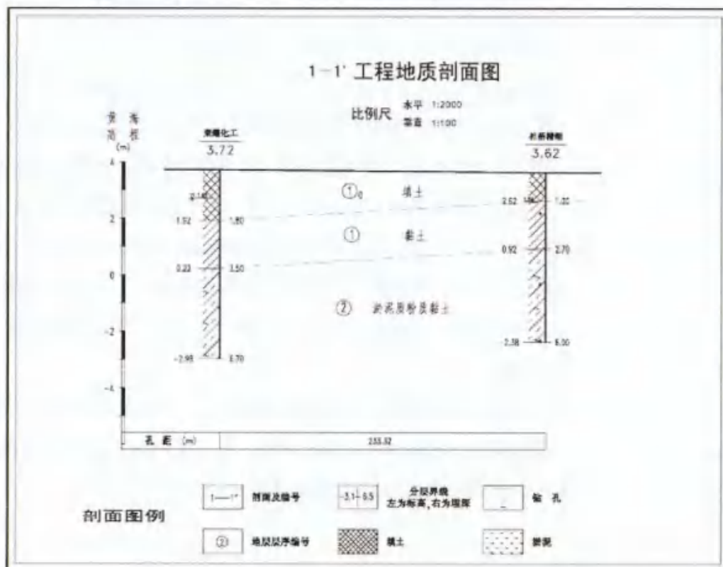
图 3.3-1 工程地质剖面图
