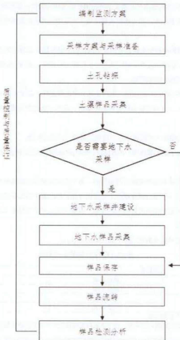
图1.3-2工作程序
