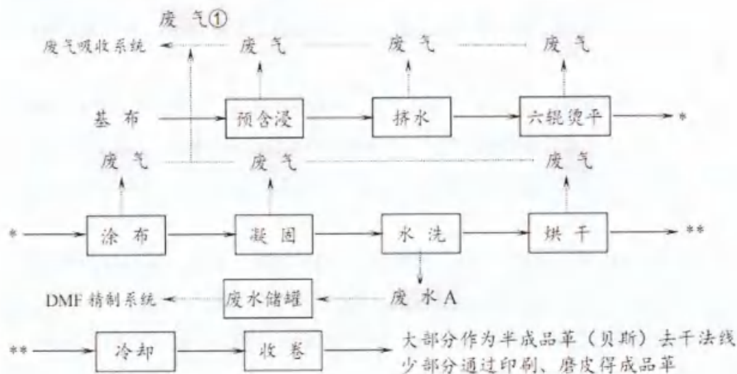
图 4.1-1 PU 合成革湿法生产线工艺流程图
