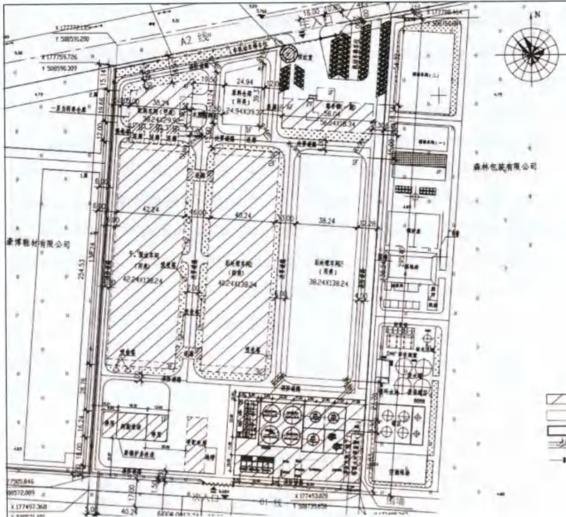
图2.2-2公司平面布置图
